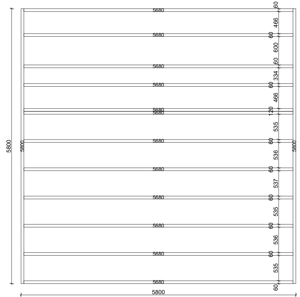
Travetti sotto pavimento 1:50
