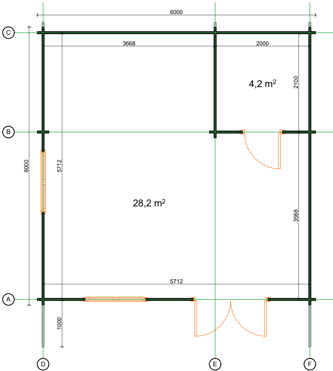
Pianta 1:50
