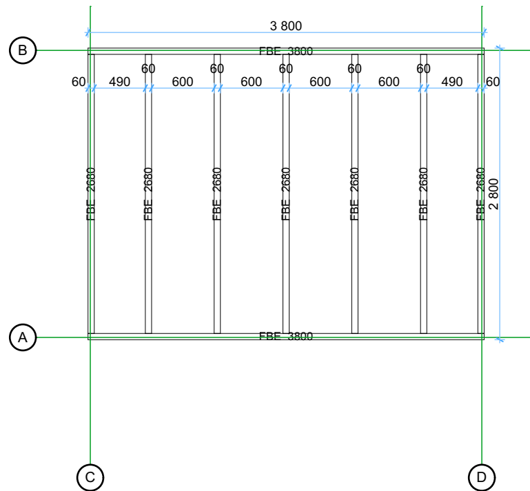
Travetti sotto pavimento
